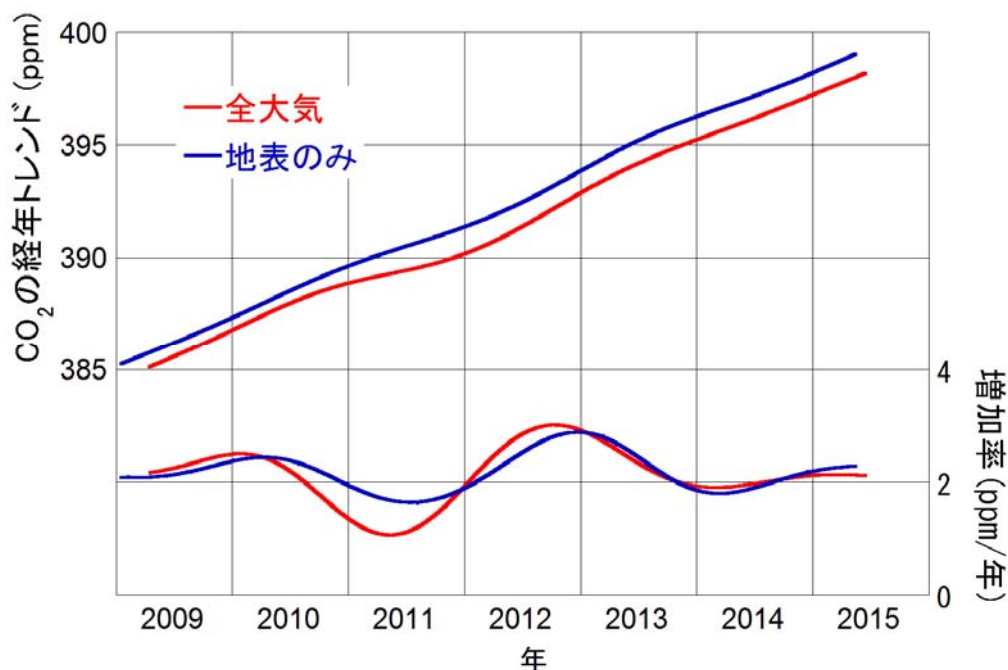
図5 二酸化炭素濃度の全大気平均（赤）と地表のみの全球平均（青）の経年トレンド（上図）と増加率（下図）
