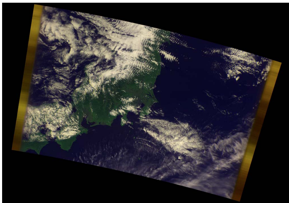
図5 TANSO-GAIレベル1B+画像の例(2009年4月23日の関東付近, 緑:バンド3, 赤:バンド2, 青:バンド1のデータを当てはめた合成画像)
